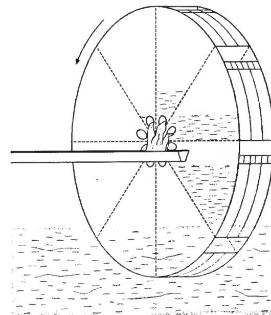
Tympanum (Rekonstruktion nach Vitr. 10,4).
